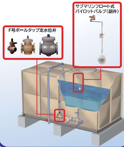
受水槽へのF号ボールタップ定水位弁設置のイメージ
